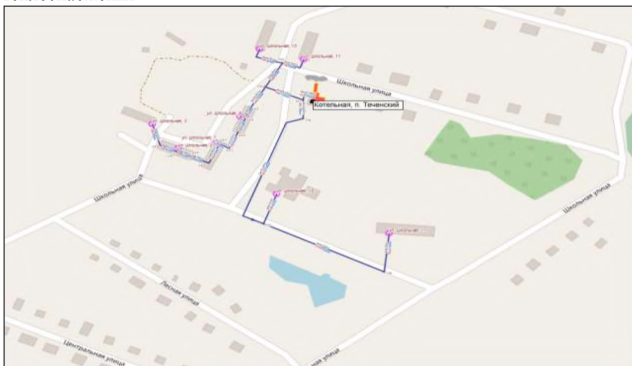
Рисунок 2.1.1. Зоны действия системы централизованного теплоснабжения
