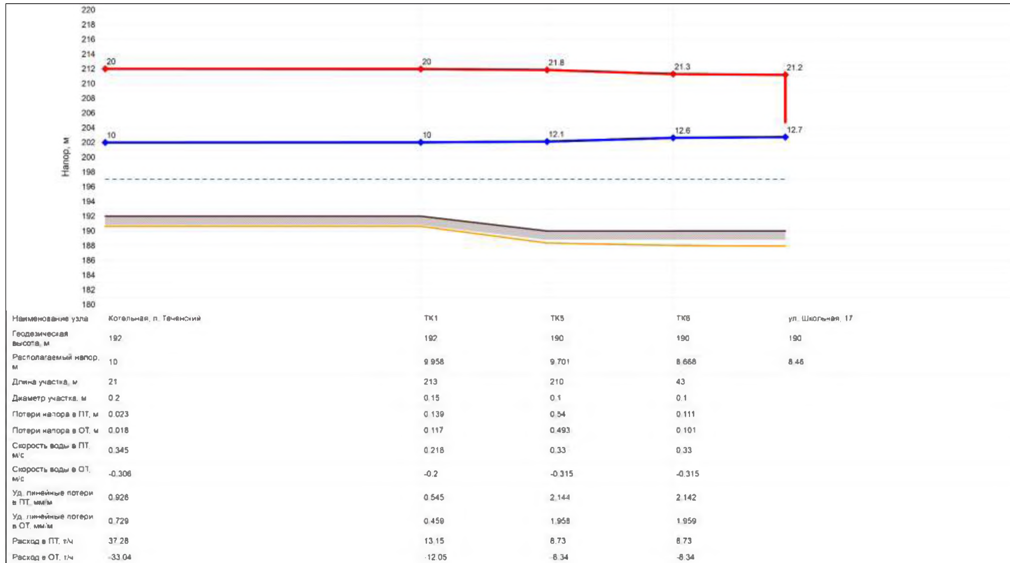
Рисунок 1.3.8.3. Пьезометрический график от Котельной, п. Теченский, ул. Школьная, 15а до ул. Школьная, 17
